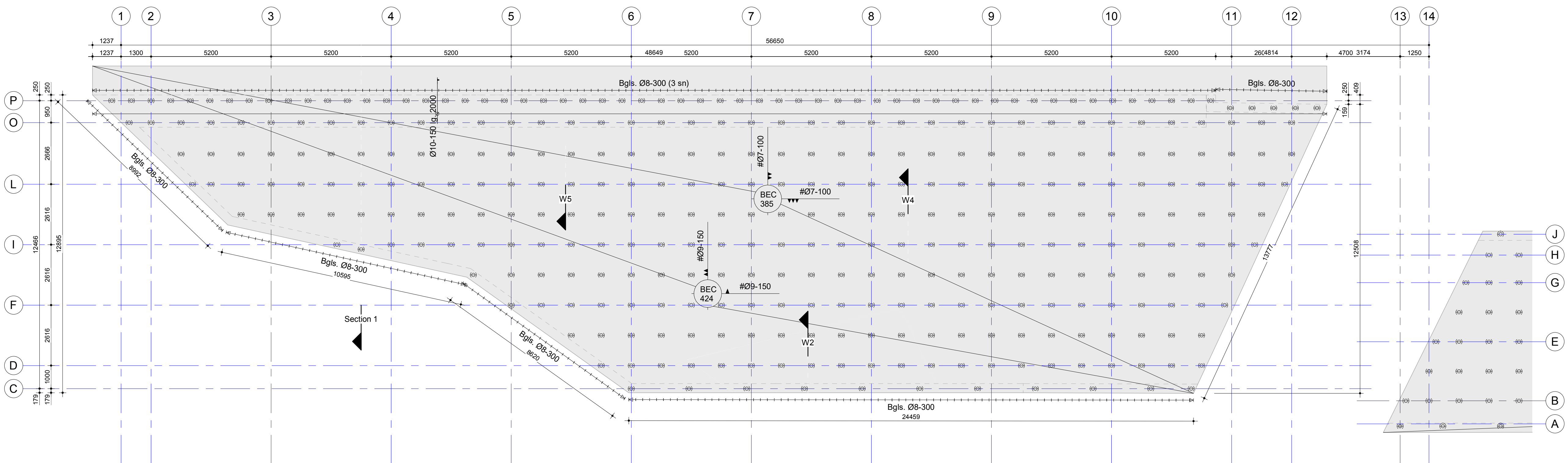
Wapening vloerplaat deel 2 1 : 100
